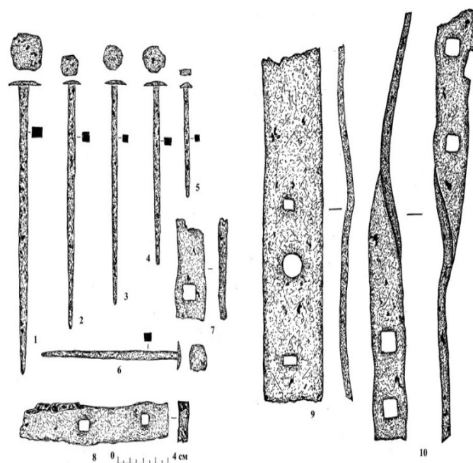
Ил. 1. Детали крепления деревянной резьбы иконостаса: гвозди 1 – 6; пластины 7-10
